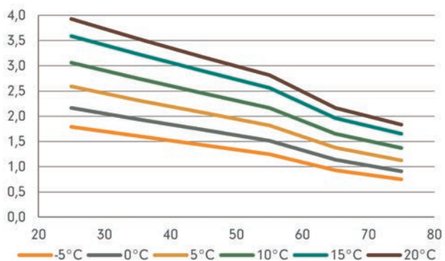
Solefluss dT4 [l/s]
