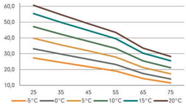
COP, 70 Hz
