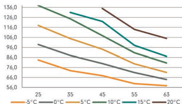
COP, 50 Hz
